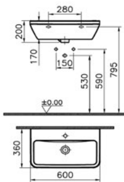
Umyvadlo compact; kód 751354
