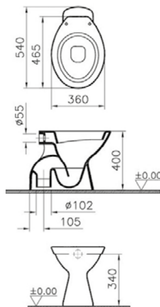
WC stojící svislý odpad kód 751347
