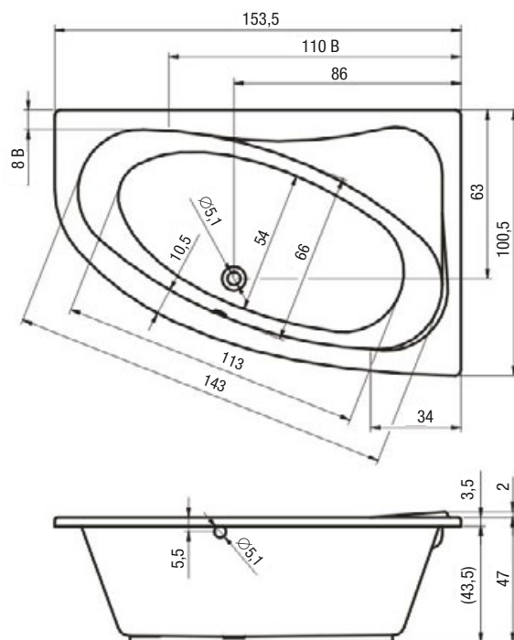
kód 293053 levá (identické rozměry kód 293054 pravá)
