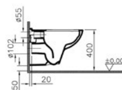
WC závěsné; kód 751355
