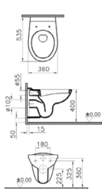
WC závěsné; kód 751342
