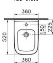
Bidet závěsný kód 751356
