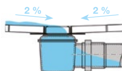
Instalace u vstupu (bez přetékání)
