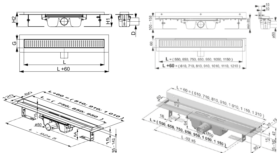
žlab sprchový kód 292731 / 292734 / 292735
