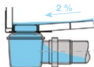
Instalace proti stěně
